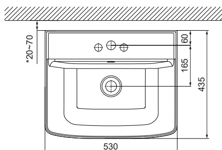
L-345VEC/AL-345VEC (3 holes)
