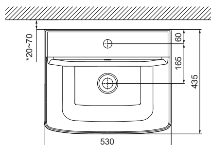
L-345VFC/AL-345VFC/CL0345F1 (1 hole)
